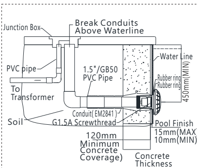
3) TOP13-EM(Concrete Pool+Liner)
