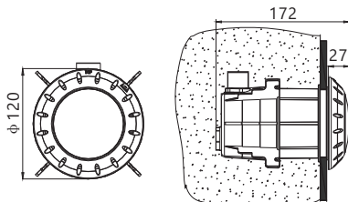
TOP13-C
