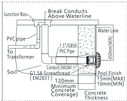
2) TOP13-EM(Concrete Pool with Conduit)
