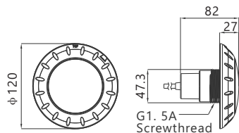
TOP13-EM
