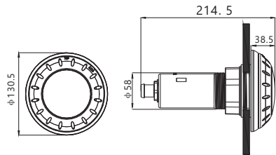
TOP13-VS
