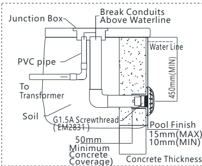
1) TOP13-EM(Concrete Pool)
