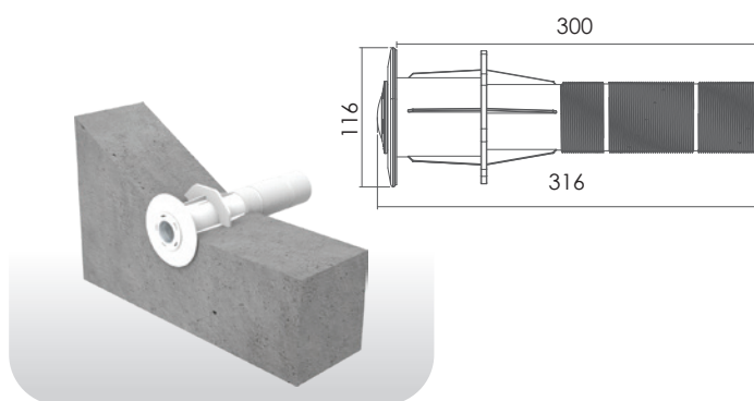
Conduits
