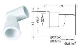
L-Type Jet Body
