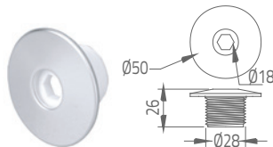
φ2" Face (Standard) Jet
